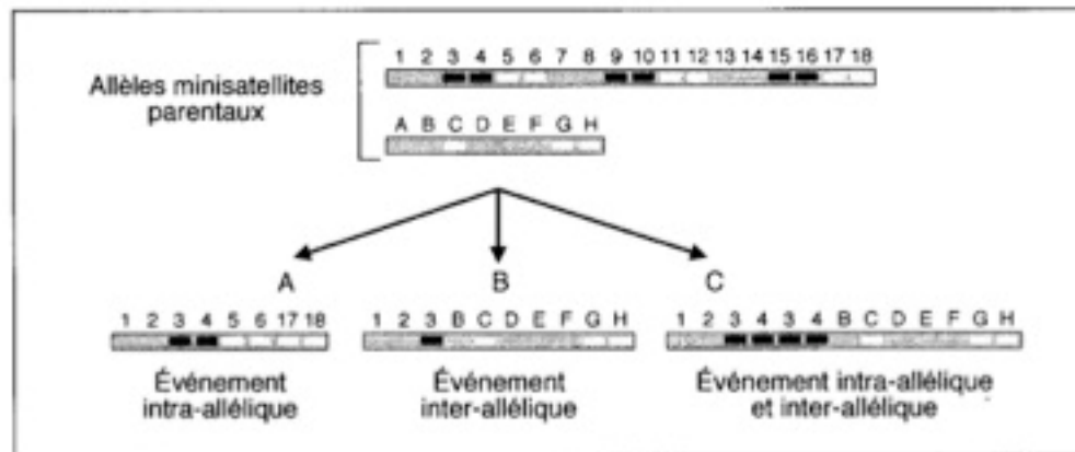
Figure 1. Exemples de réarrangements survenus au niveau de la répétition minisatellite après les divisions méiotiques dans la levure. Chaque motif minisatellite est représenté par un rectangle. Les polymorphismes entre les différents motifs composant le minisatellite sont schématisés par les différentes couleurs des rectangles (gris, blanc ou rouge). Les motifs du premier allèle minisatellite parental sont numérotés de 1 à 18 et ceux du second allèle parental sont notés de A à H. À l'issue de la méiose, plusieurs types d'événements sont obtenus. A. Événements intra-alléliques. L'exemple schématisé correspond à une délétion intra-allélique des motifs 7 à 16. B. Événements inter-alléliques. L'exemple schématisé correspond à une fusion des motifs 1 à 3 du premier allèle parental avec les motifs B à H du second allèle parental. C. Événements complexes. L'exemple schématisé correspond à un événement intra-allélique avec une duplication des motifs 3 et 4 du premier allèle parental et un événement inter-allélique où les motifs 1 à 4 du premier allèle parental sont joints aux motifs B à H du second allèle parental.
